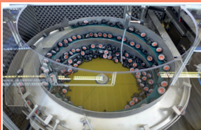
Komponentenzuführung
