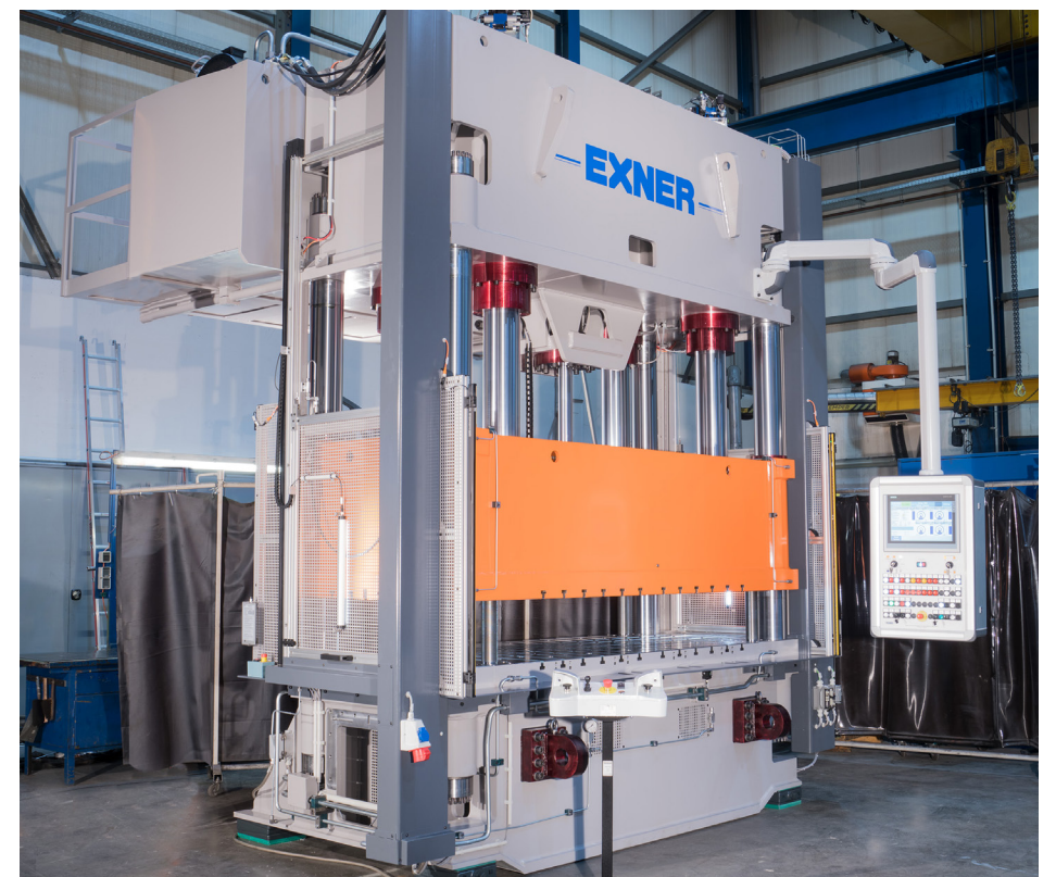
Werkzeugprobierpresse PG-4 „four drive axes“ 800 – 10.000 kN
